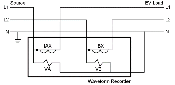
Fig. 1. Metering diagram
