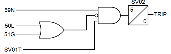
Fig. 8. 3V0 OPD Scheme
