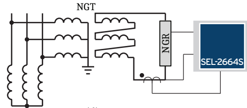
(d) Injecting current via broken-delta winding of VT
