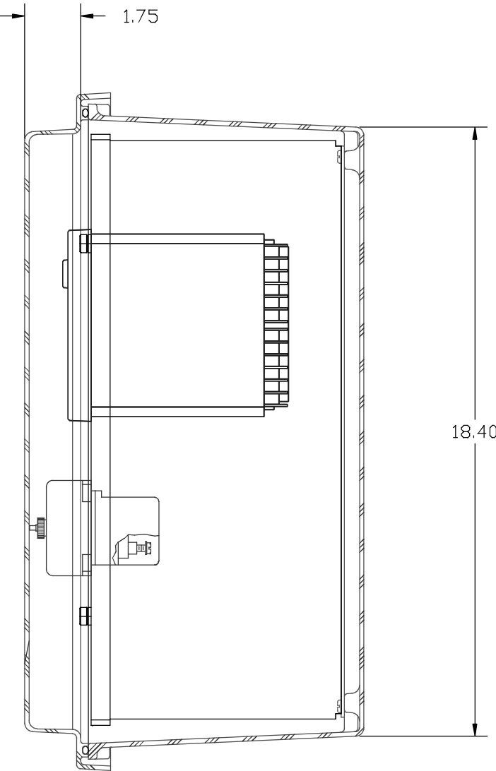
SECTION A-A
